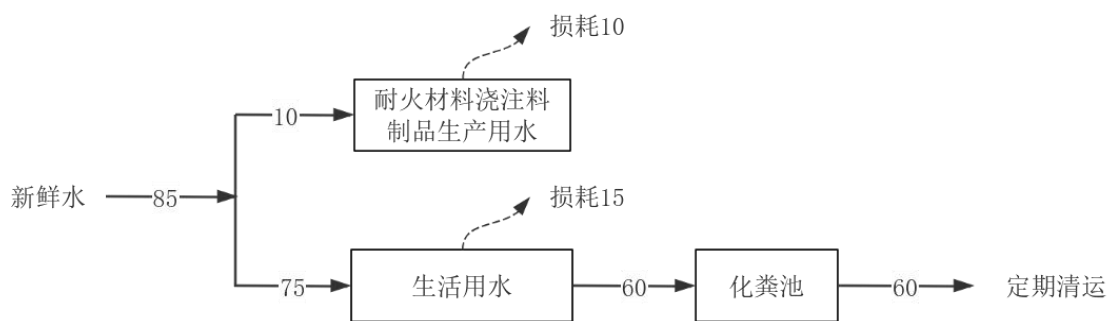
图2-1 项目水平衡图 (m³/a)
