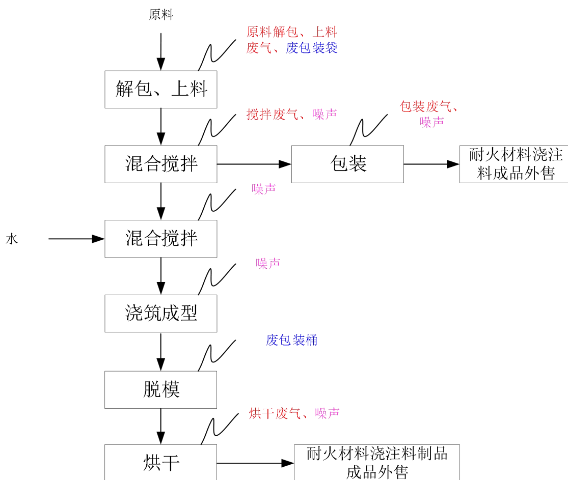
图2-2 项目生产工艺及产污环节图
